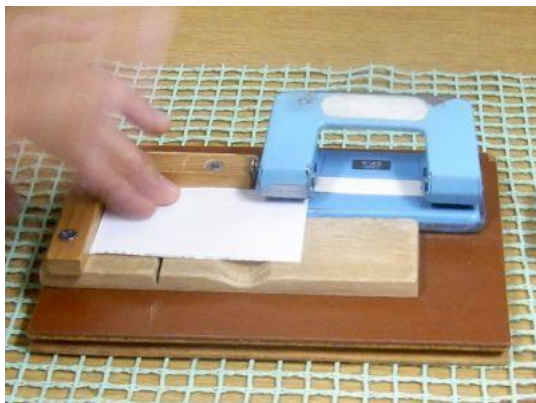
【上下判別のくぼみを入れる治具】
